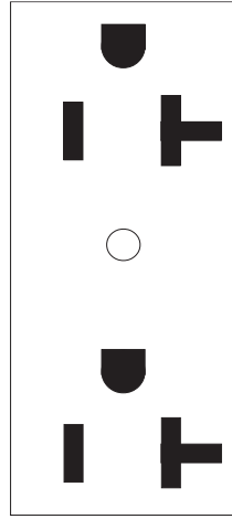
5-20 DUPLEX 20A - 125 Volt Straight Blade #5
