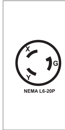
L6-20 SINGLE 20A - 250 Volt Twist Lock #10
