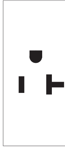
5-20 SINGLE 20A - 125 Volt Straight Blade #6
