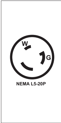
L5-20 SINGLE 20A - 125 Volt Twist Lock #9
