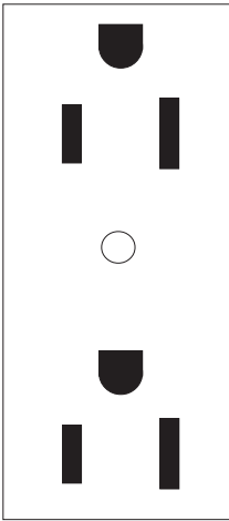
5-15 DUPLEX 15A - 125 Volt Straight Blade #2
